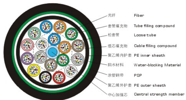
光缆结构图 Cable Structure
